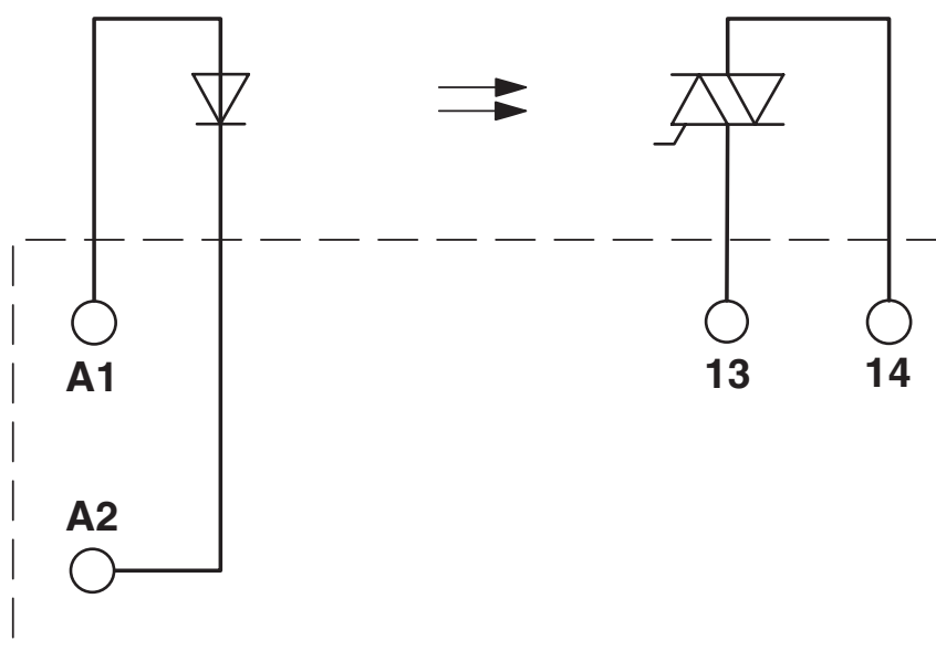
Diagrama eléctrico
