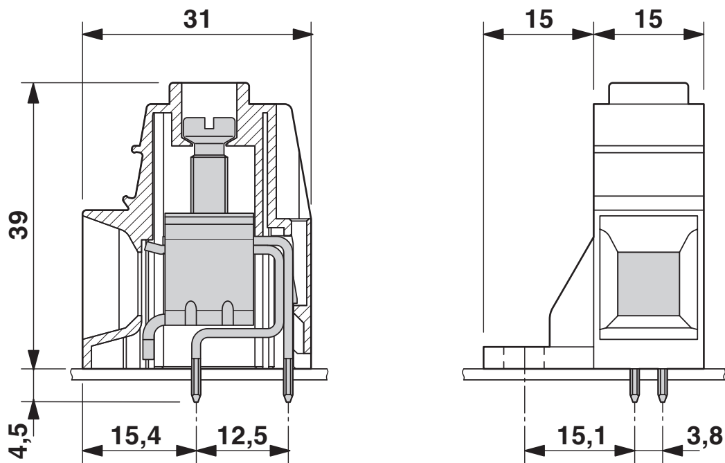
Maßzeichnung
