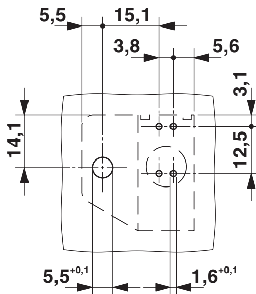
Bohrplan/Lötpadgeometrie
