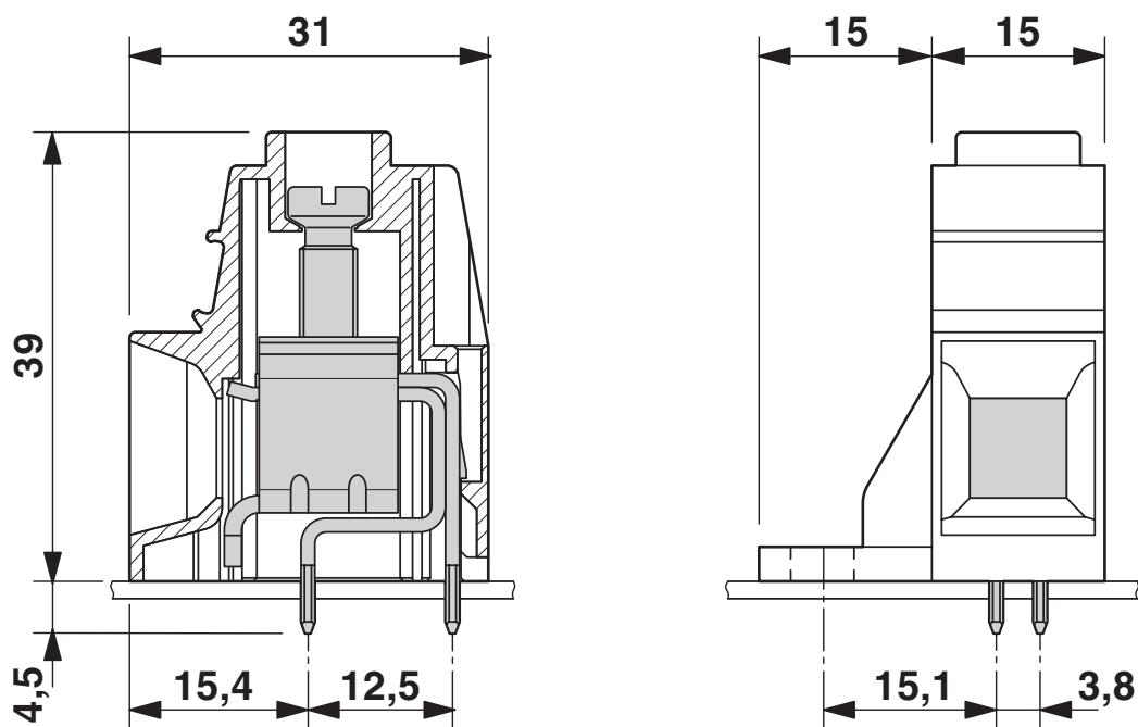
Dessin coté
