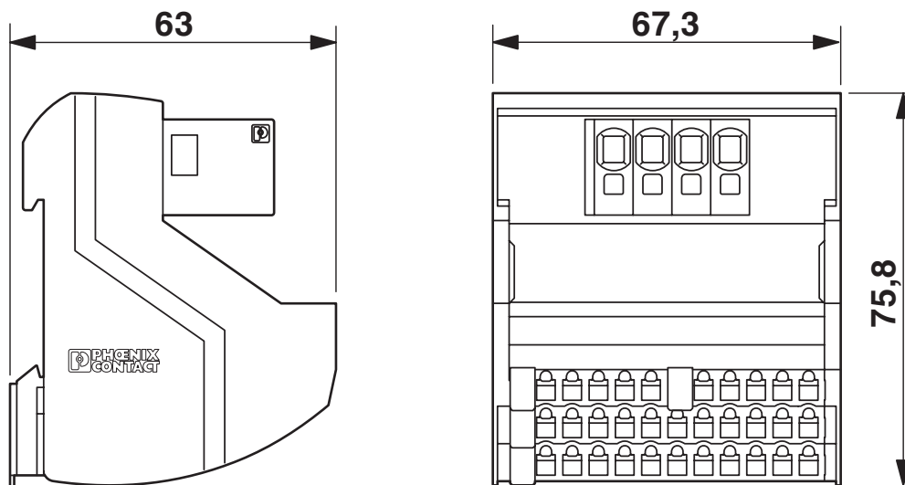
Maßzeichnung
