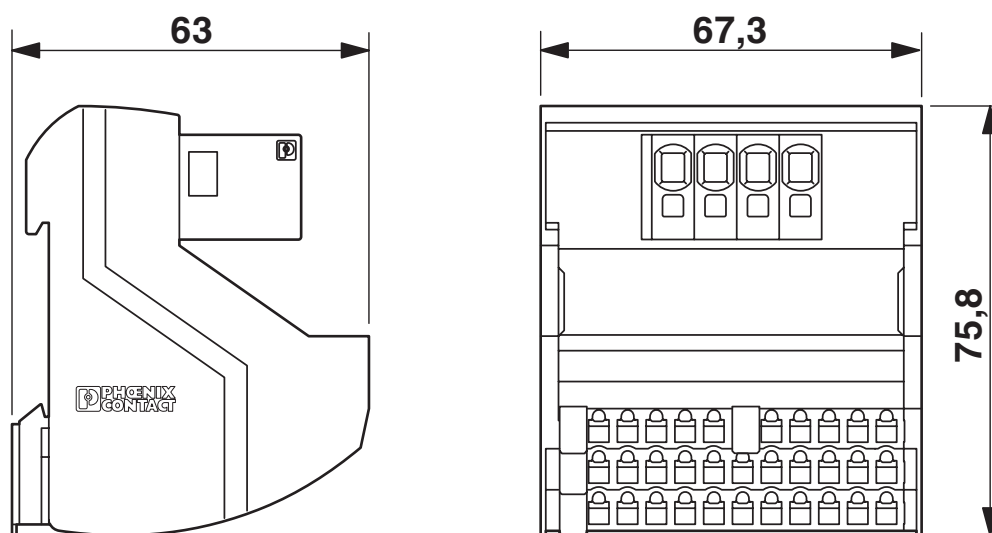
Dessin coté
