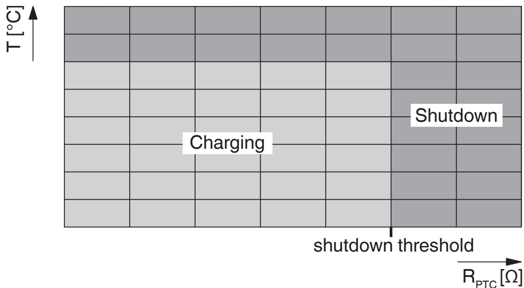
Schemazeichnung
