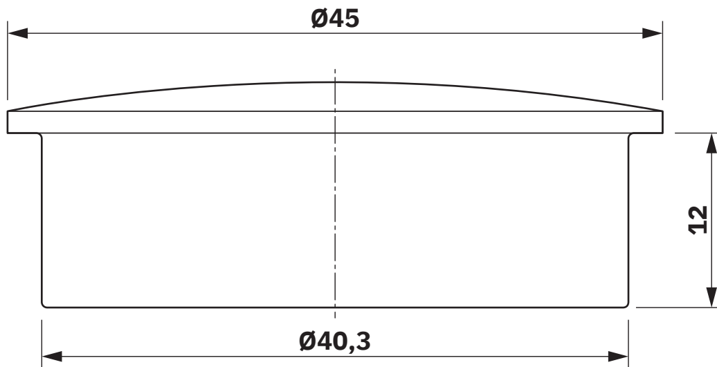
Maßzeichnung
