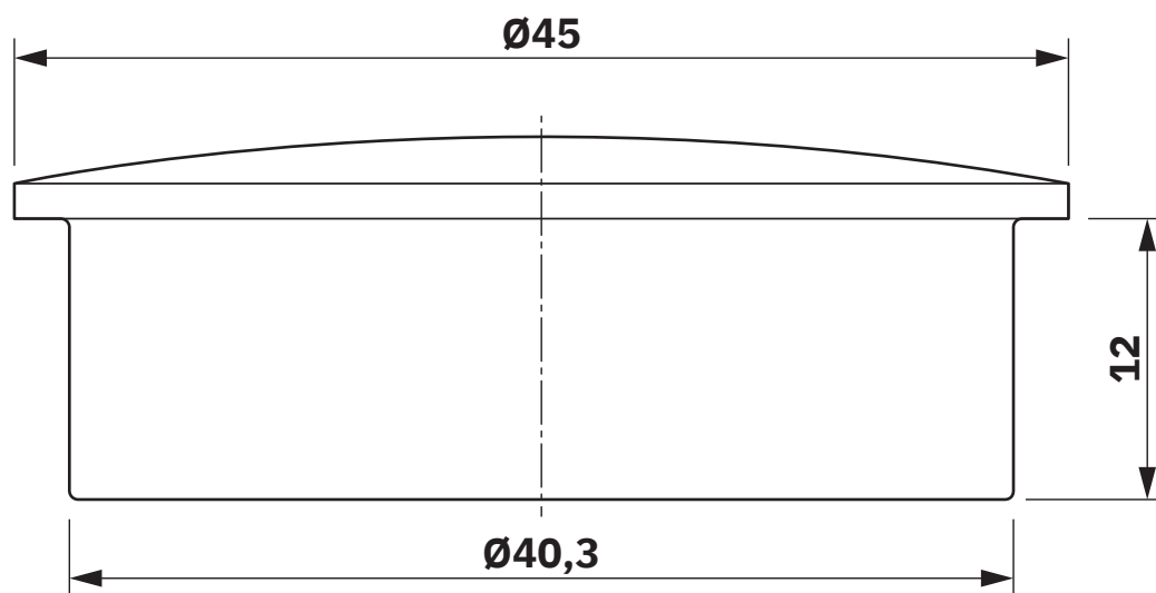
Dessin coté
