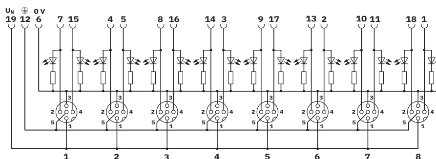
Diagrama eléctrico
