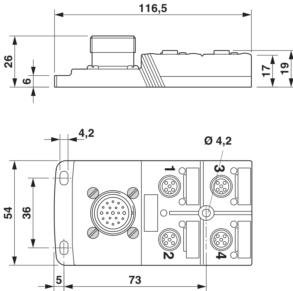
Dessin coté
