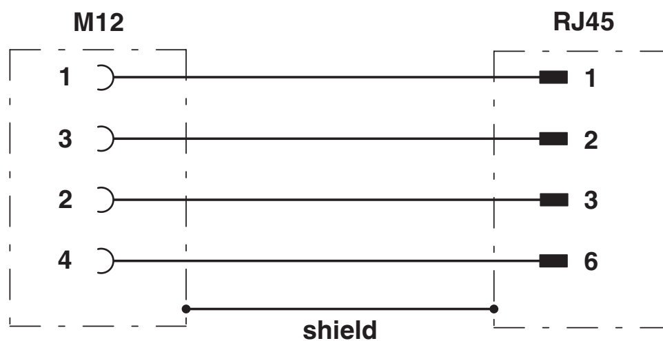
Diagrama eléctrico
