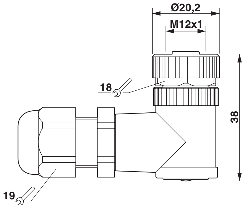
Maßzeichnung
