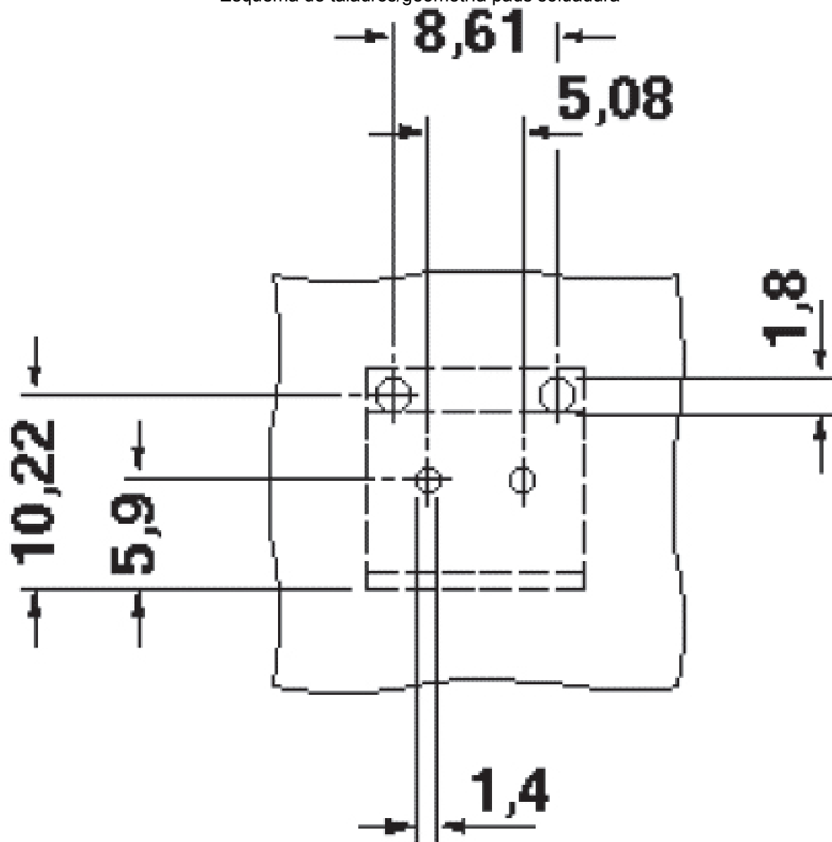
Esquema de taladros/geometría pads soldadura
