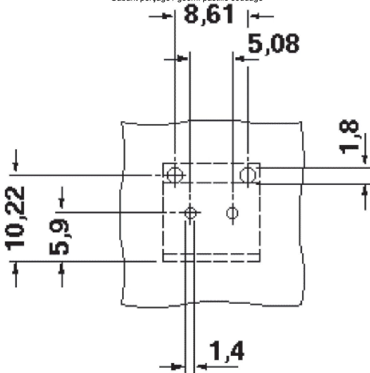
Gabarit perçage / géom. pastille soudage
