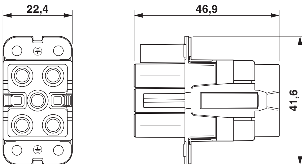
Dessin coté
