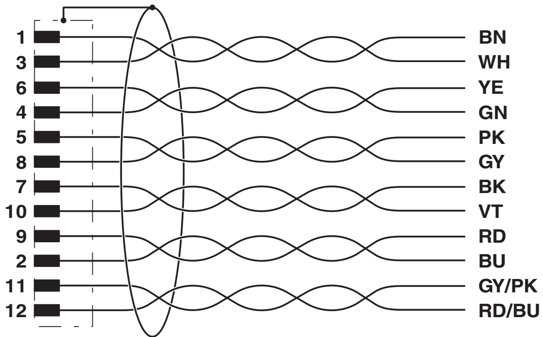
Schaltplan
