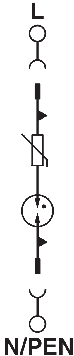
Schaltplan
