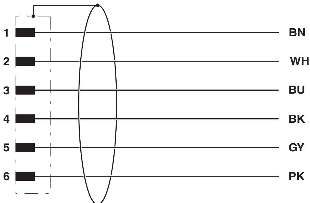
Diagrama eléctrico
