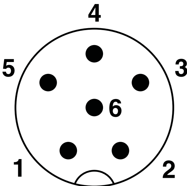
Plano esquemático
