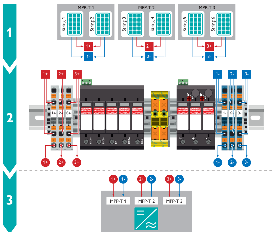
Schéma de l'application schématique
