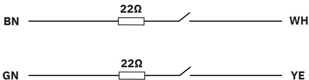
Diagrama eléctrico
