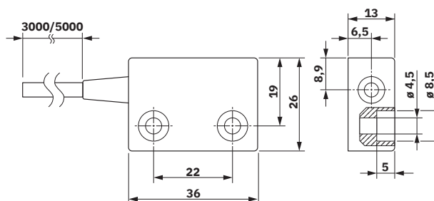
Dessin coté
