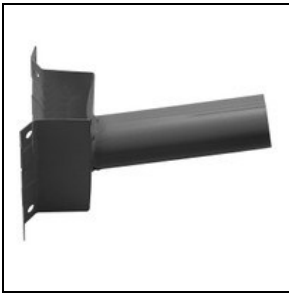
14077796 Soporte de acero pintado en Electroforesis con polvo de poliéster para las instalaciones en una esquina o en la pared ■ AN-g6 / Antracita metalizado
