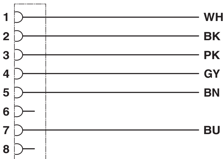
Schaltplan
