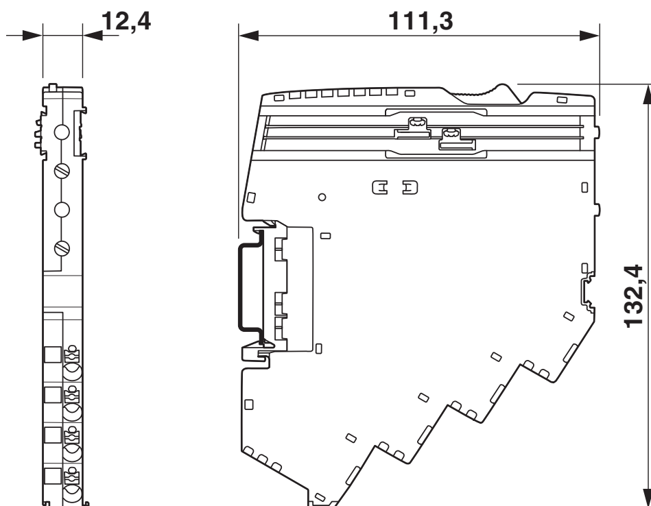
Dessin coté
