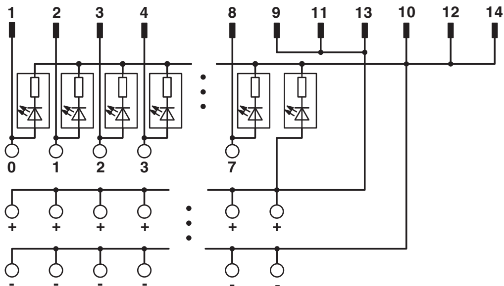
Diagrama eléctrico
