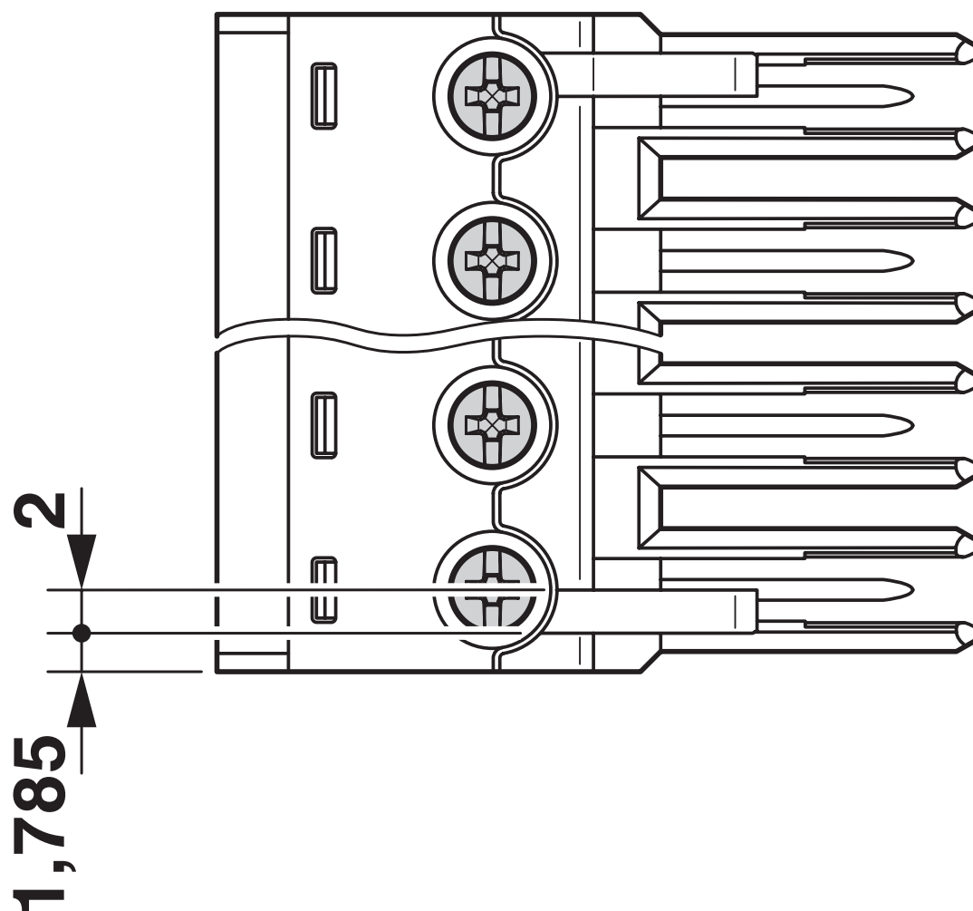
Maßzeichnung
