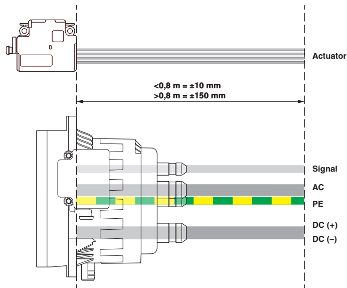
Dessin coté
