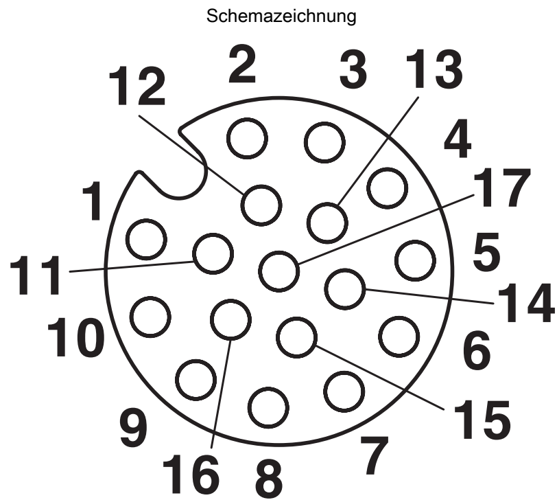
Polbild Buchse M12, 17-polig, A-kodiert, Ansicht Buchsenseite
