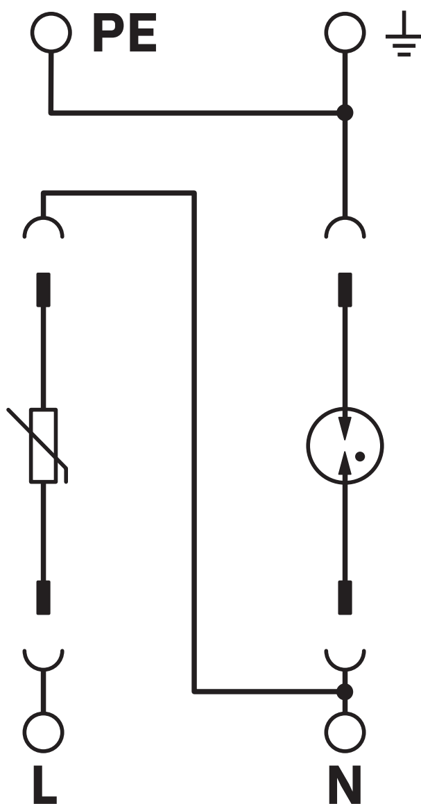
Diagrama eléctrico
