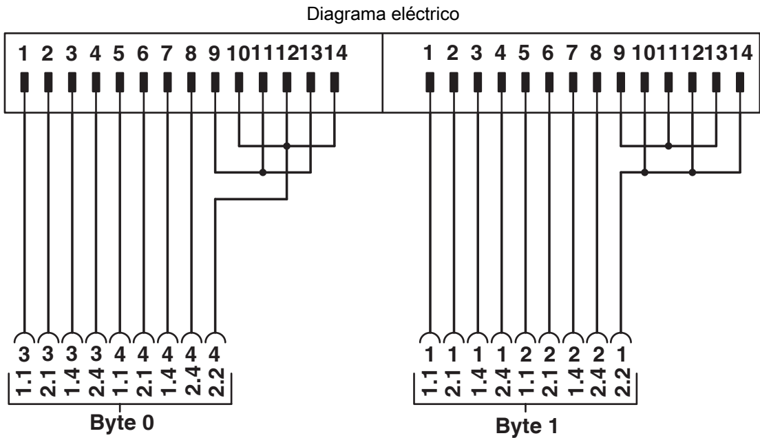
Esquema de conexiones FLKM 14-PA-INLINE/OUT16
