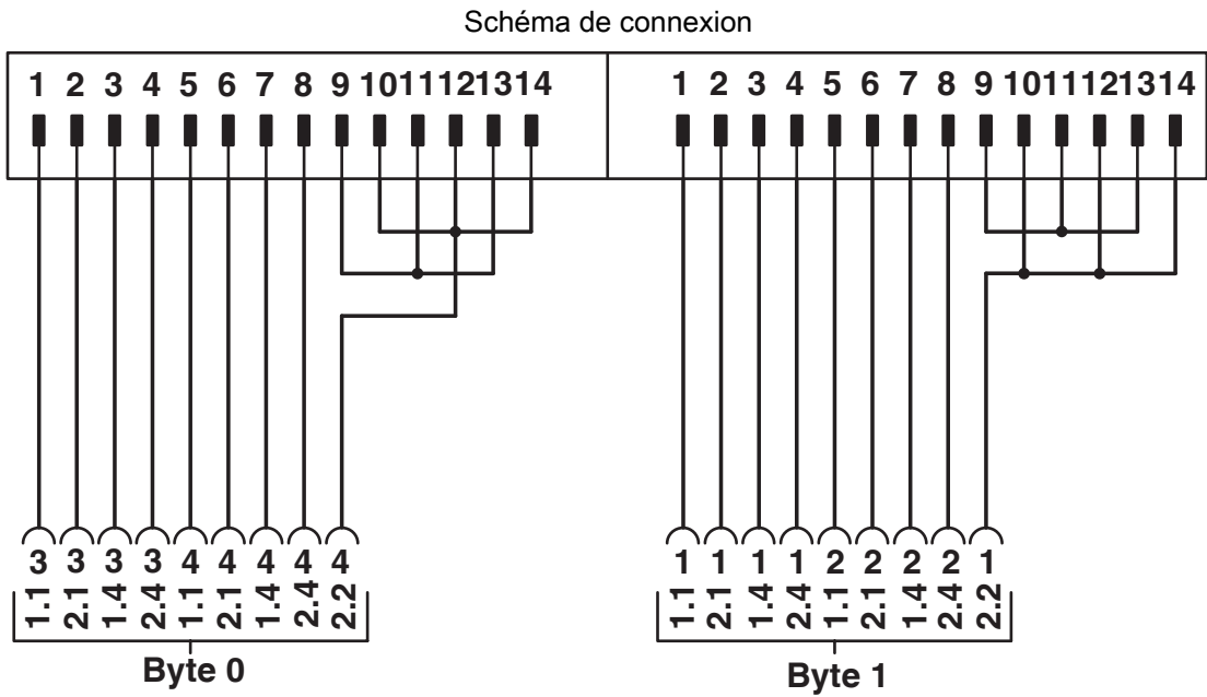
Schéma des connexions FLKM 14-PA-INLINE/OUT16
