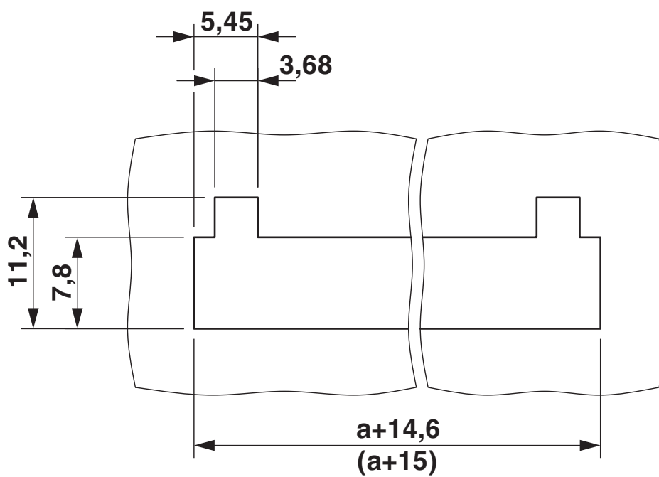
Maßzeichnung
