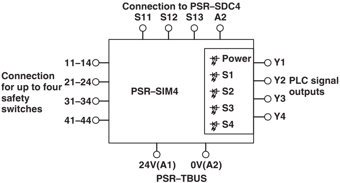
Diagrama eléctrico
