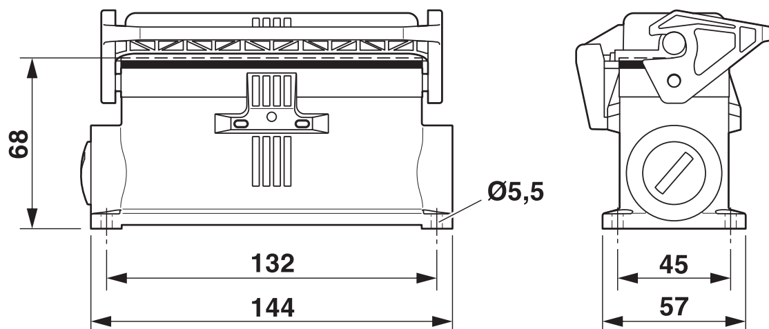
Dessin coté
