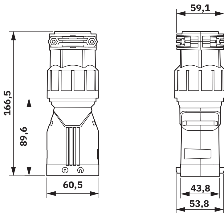
Dessin coté
