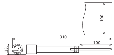
Maßbild S 100 ZK MS
