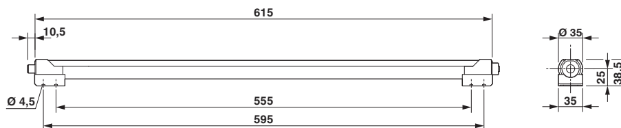
Maßzeichnung
