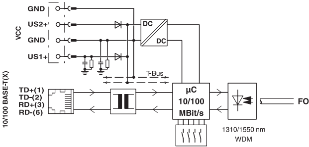
Schéma fonctionnel
