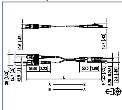
Maßzeichnung
