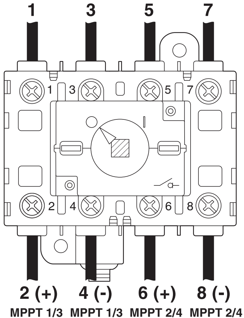
Anschlusszeichnung
