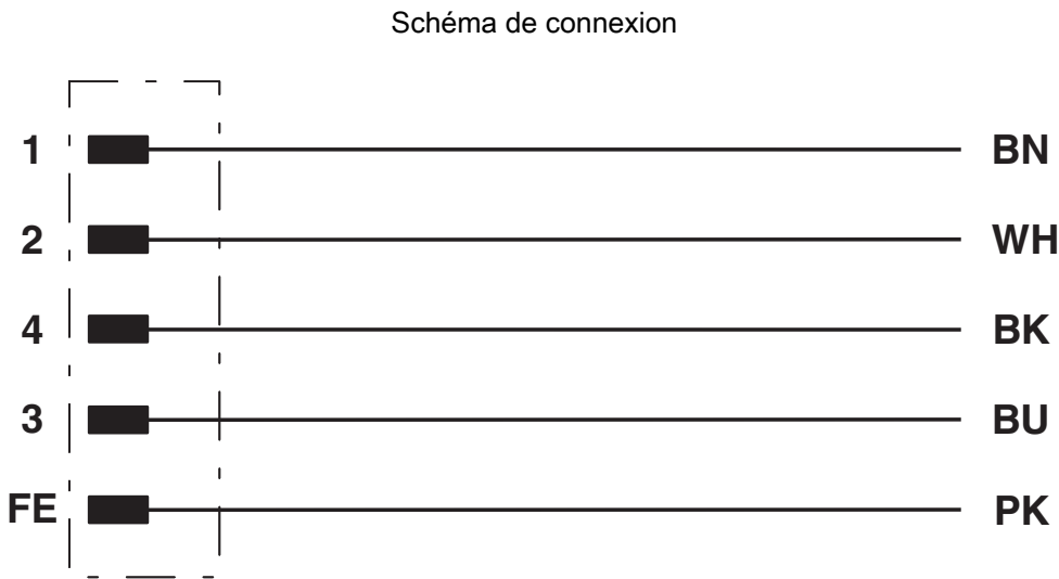
Affectation des contacts du connecteur mâle M12
