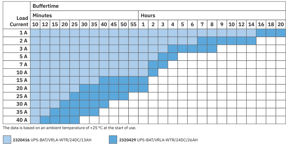
Durées d'autonomie de QUINT DC UPS et du module de batterie VRLA-WTR
