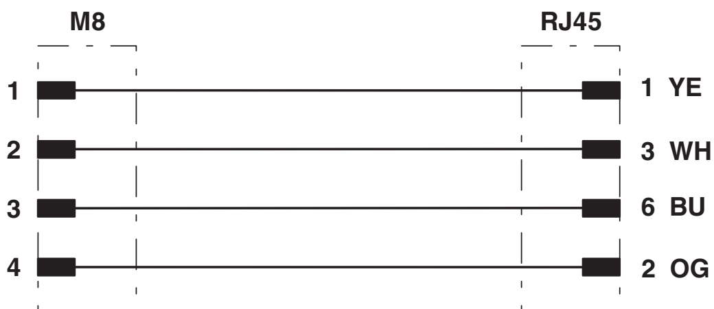
Kontaktbelegung des M8- und RJ45-Steckers
