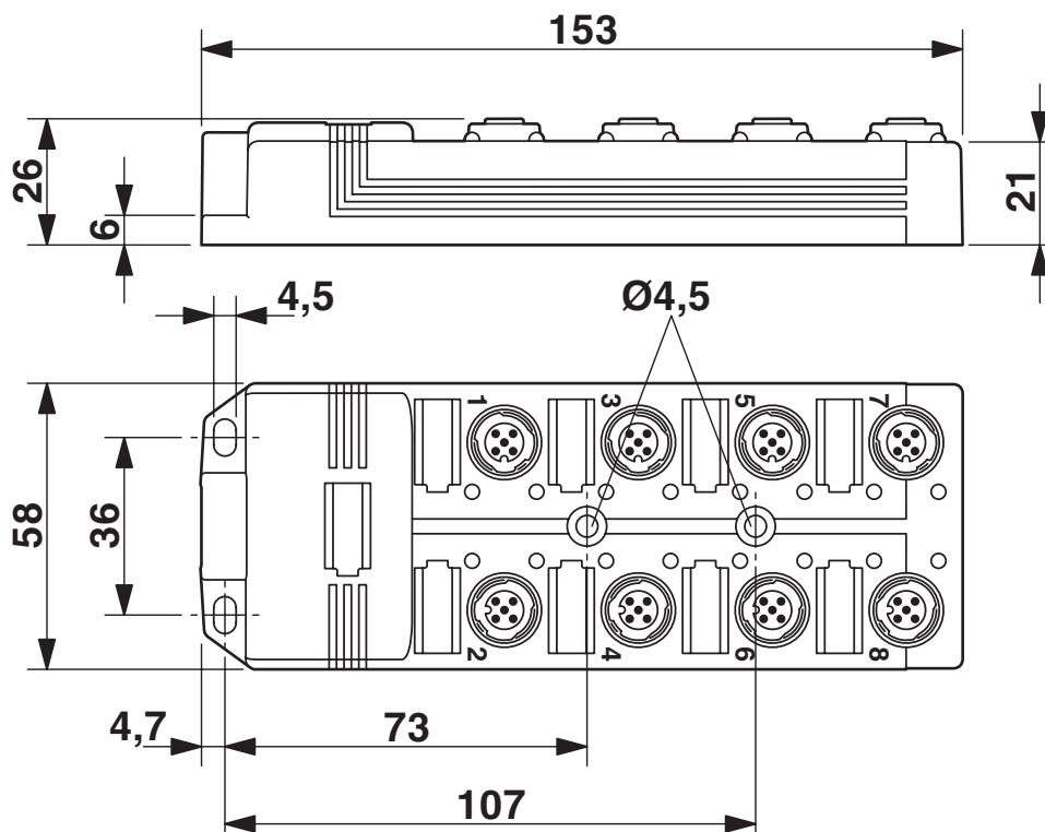
Dessin coté
