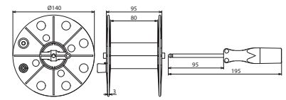
Maßbild DH K 80 BB ASG L
