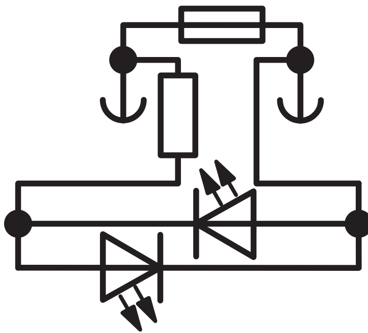
Schéma de connexion
