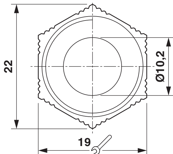
Dessin coté
