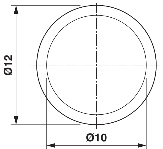
Dessin coté
