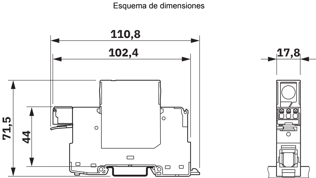
Plano esquemático
