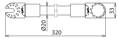
Maßbild ISV 320 ZK MS
