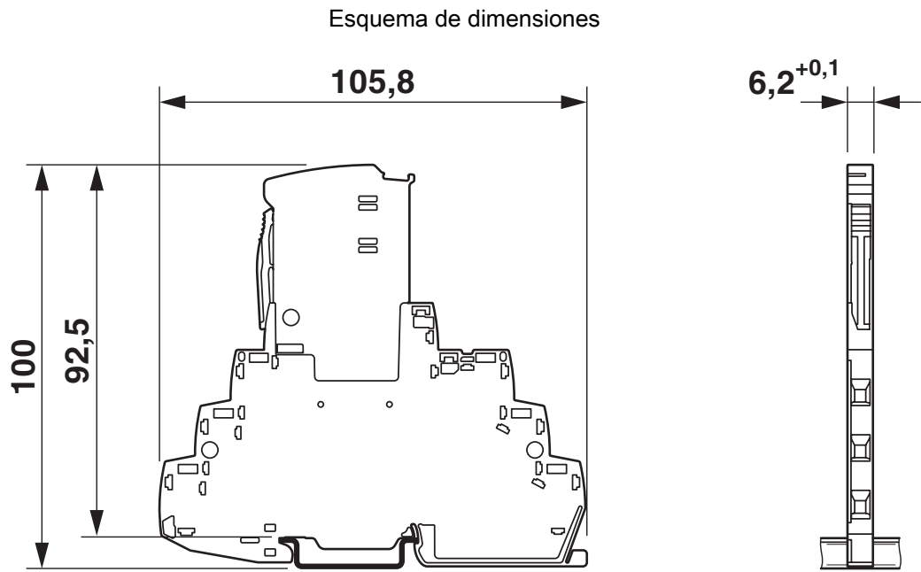
Plano esquemático
